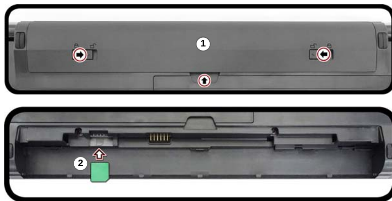
Figura 17 - Rimozione della batteria e inserimento della carta USIM
