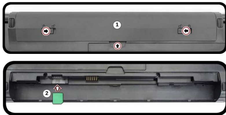
Abb. 17 - Herausnehmen des Akkus und einsetzen der USIM-Karte
