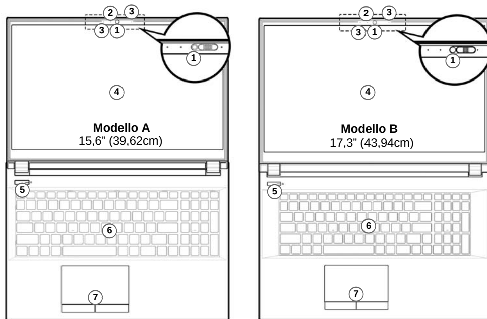
Figura 2 - Vista anteriore con lo schermo aperto
