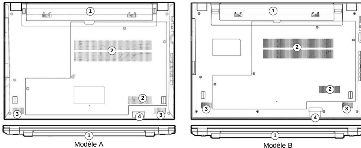
Figure 6 Vues de dessous et arrière
