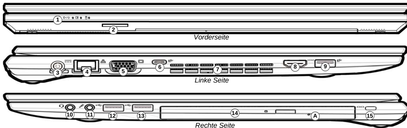
Abb. 5 - Ansicht von vorne, links und rechts (Modell B)
