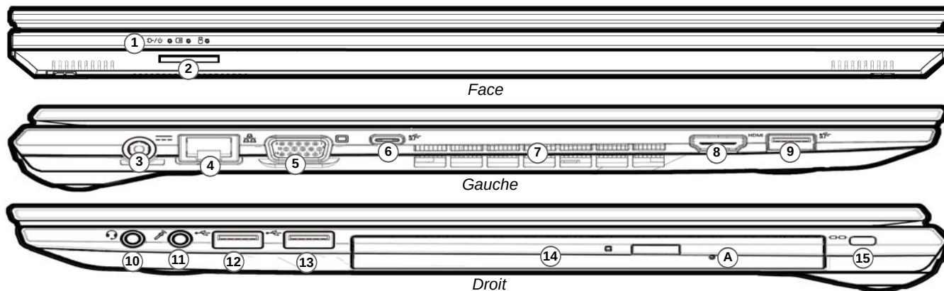
Figure 5 - Vues de face, gauche et droite (Modèle A)
