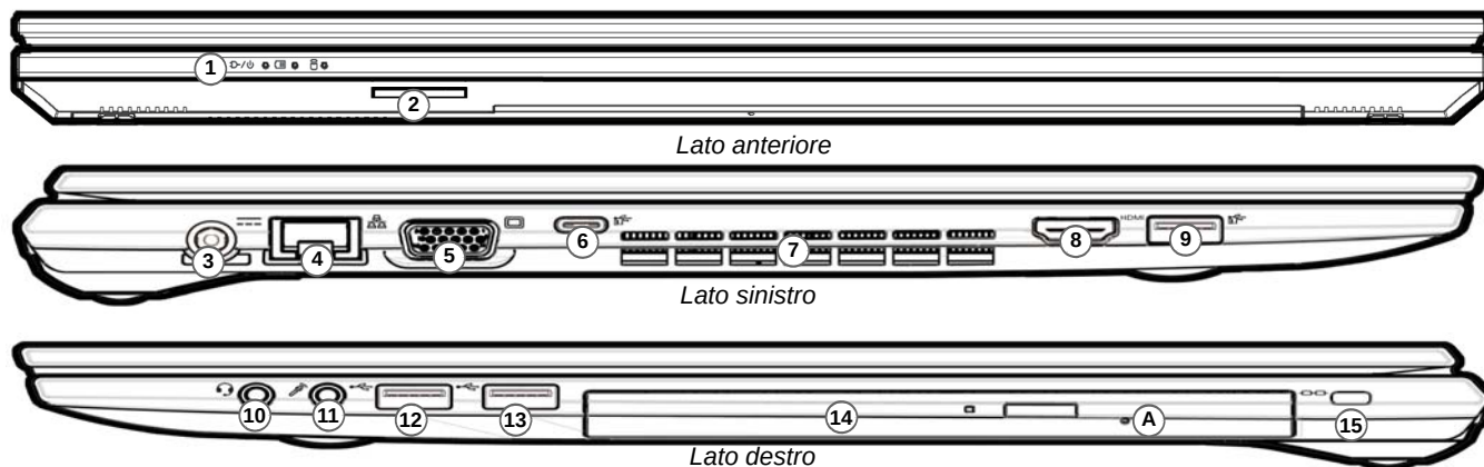
Figura 5 - Vista anteriore, sinistra e destra (Modello B)
