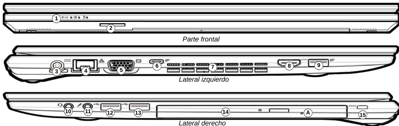
Figura 5 - Vistas frontal, izquierda y derecha (Modelo B)
