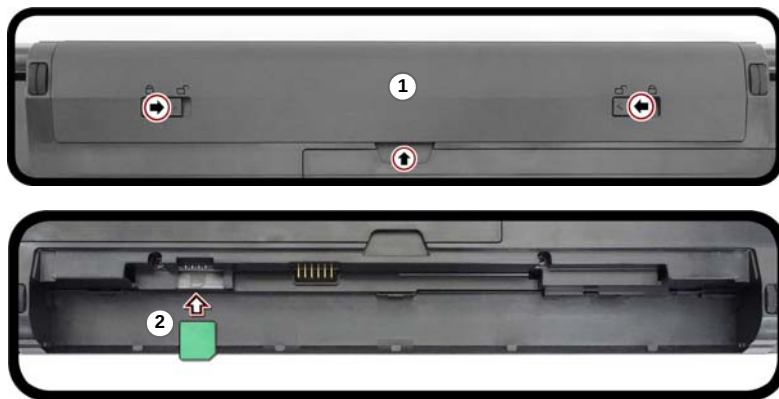
Figure 17 - Retirer la batterie et insérer la carte USIM
