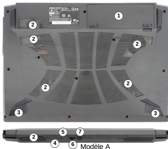
Figure 6 Vues de dessous et arrière
