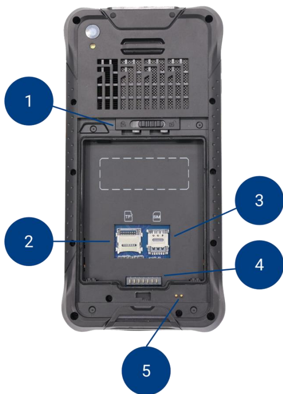
Abbildung 2 Pokini Tab FS6B, innenliegende Interfaces
